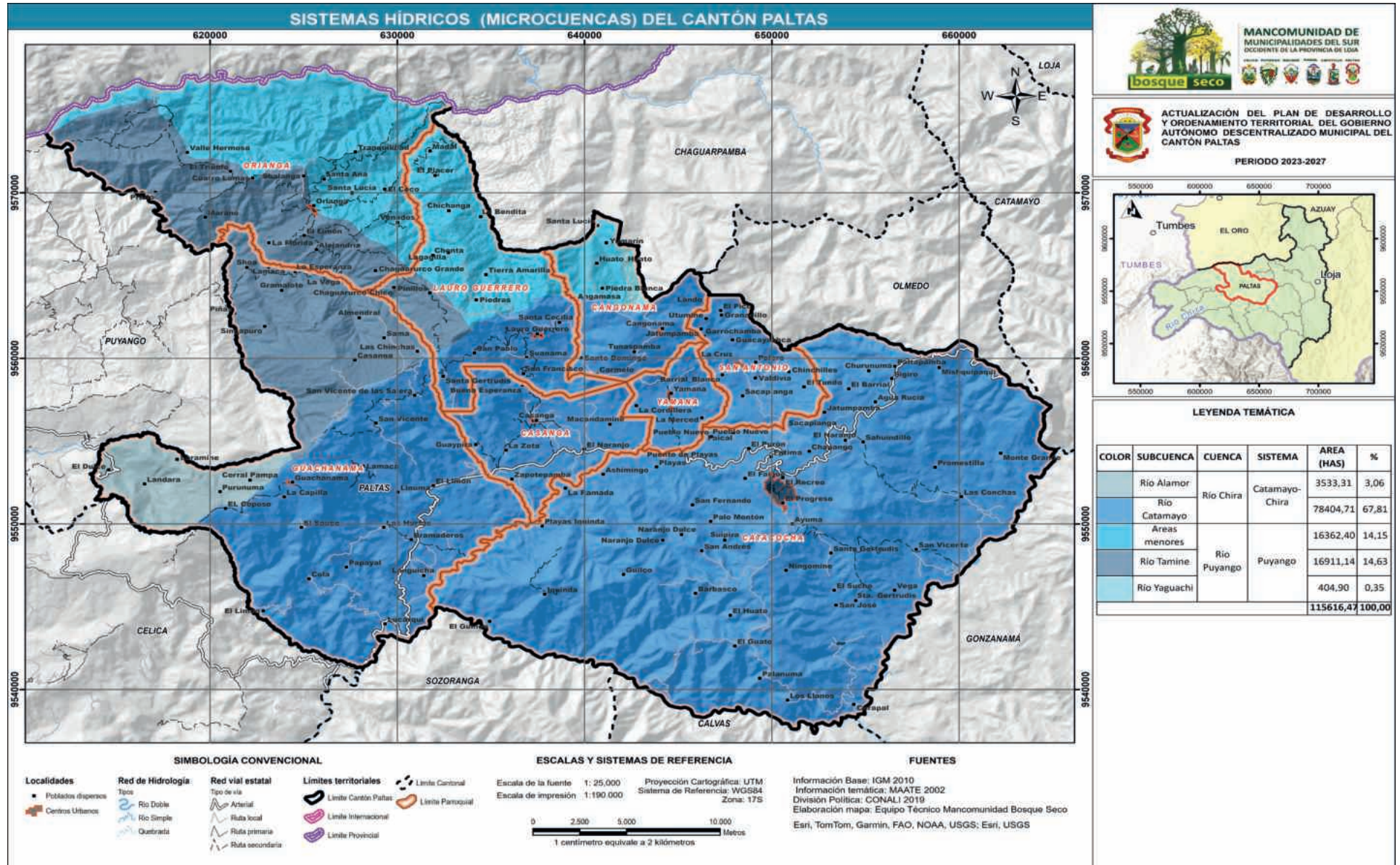
Mapa 3. Sistemas hídricos del cantón Paltas
