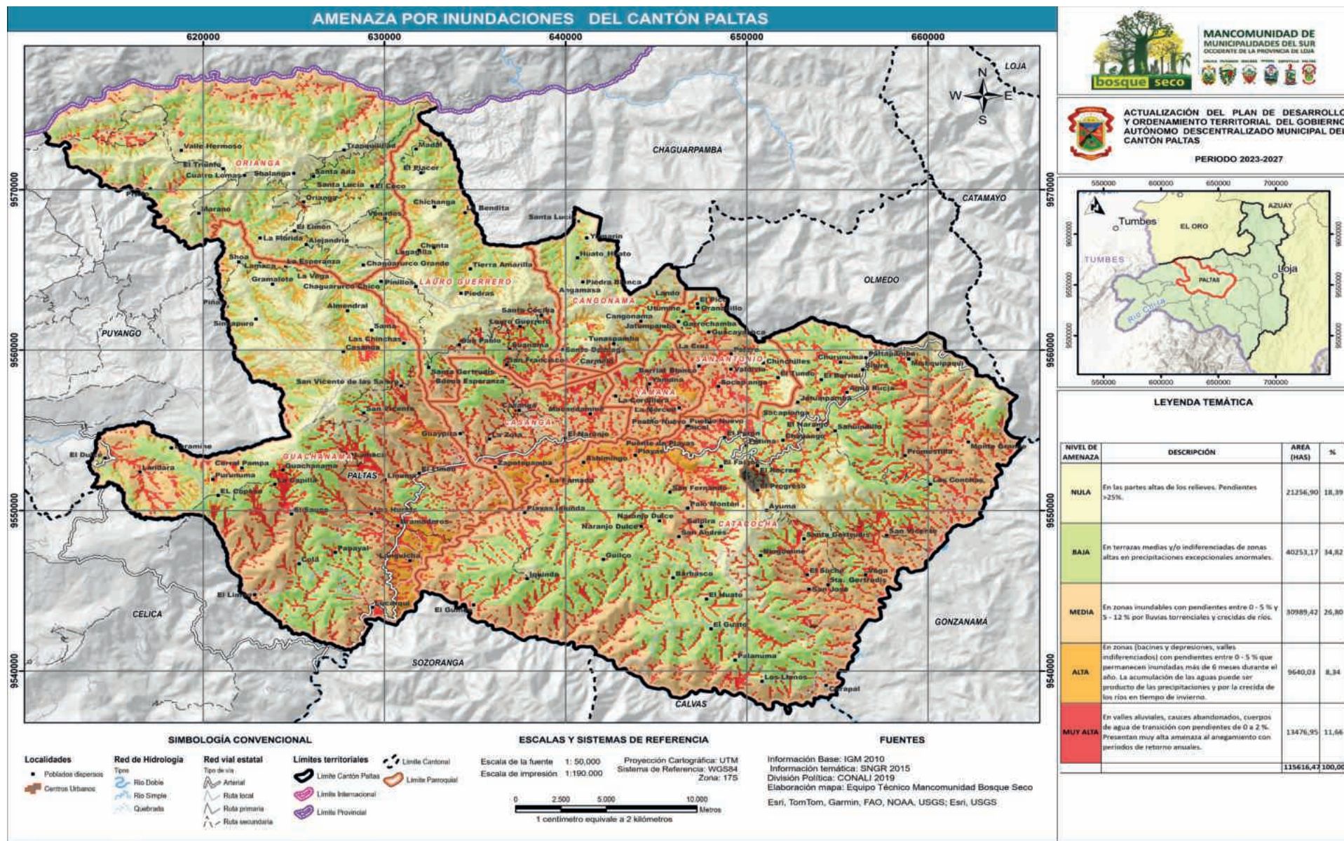
Mapa 12. Amenaza por inundaciones del cantón Paltas
