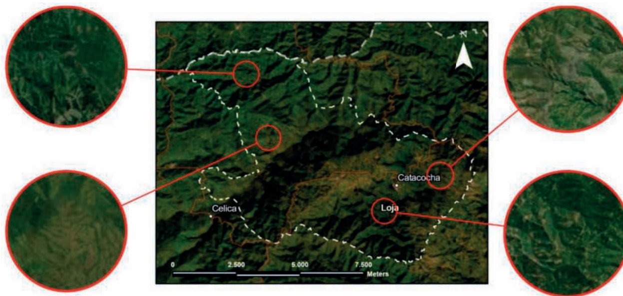
Figura 4. Fragmentación de los ecosistemas del cantón Paltas
