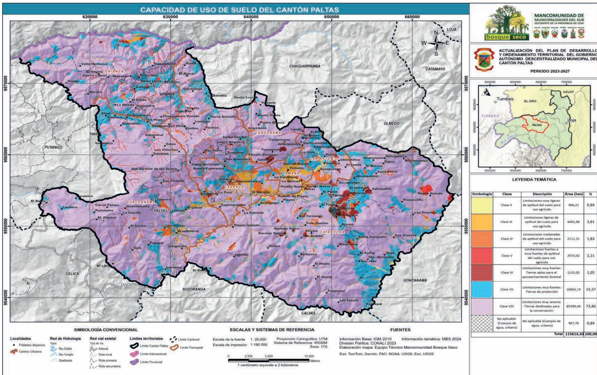
Mapa 7. Capacidad de Uso de Suelo del cantón Paltas
