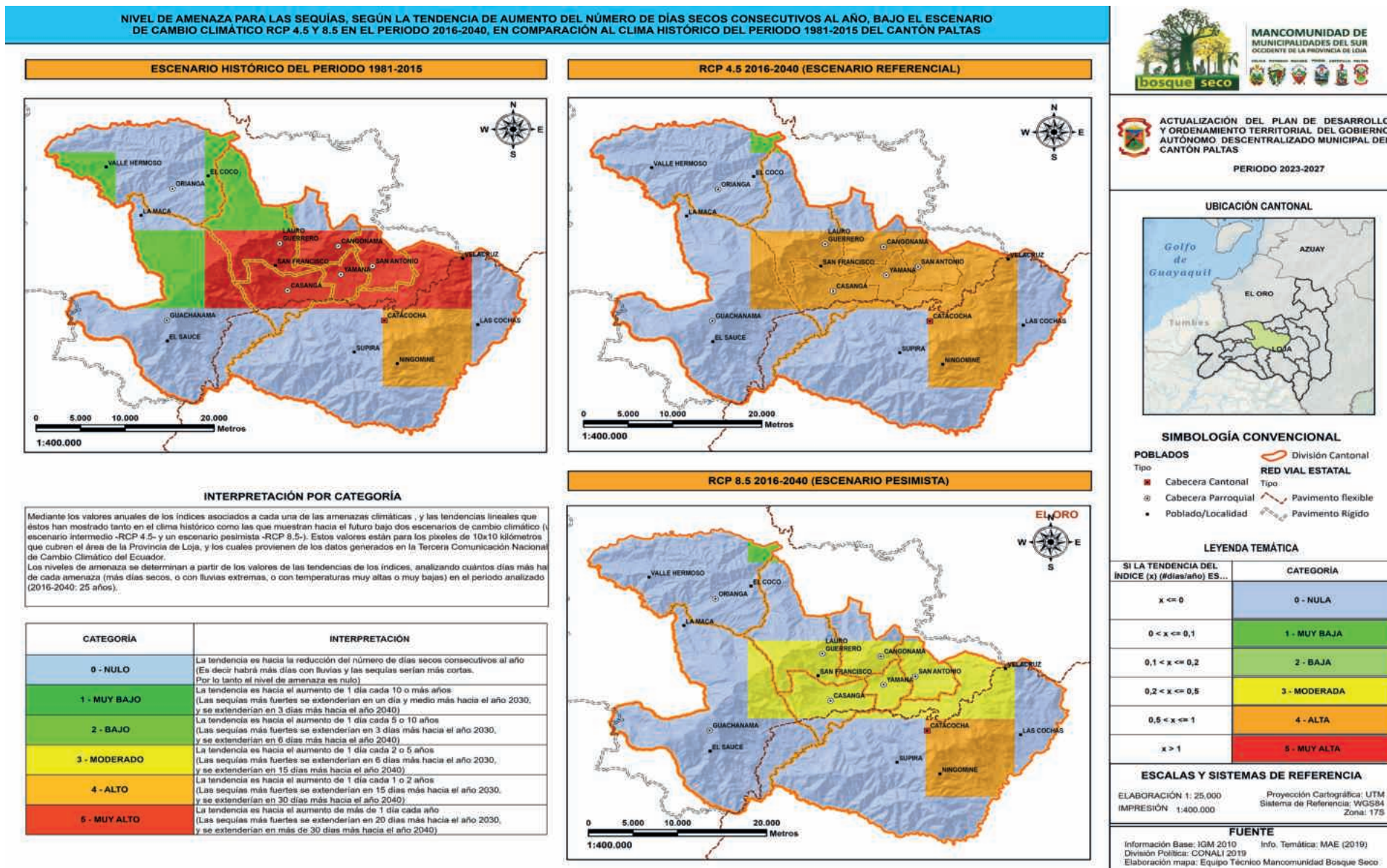
Mapa 14. Escenario de sequías del cantón Paltas.
